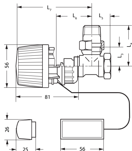
Угловой вертикальный клапан с термостатическим элементом RA2992
